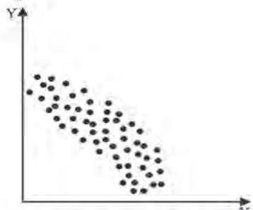
चित्र 6.7 ऋणात्मक गैर-रेखीय संबंध
